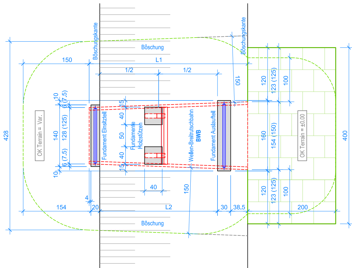
GRUNDRISS 1:50
