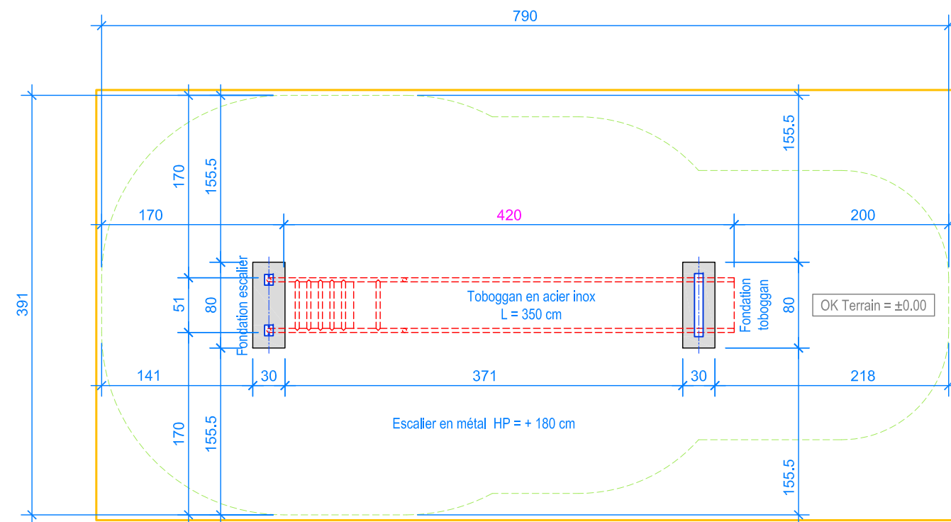
PLAN 1:50
