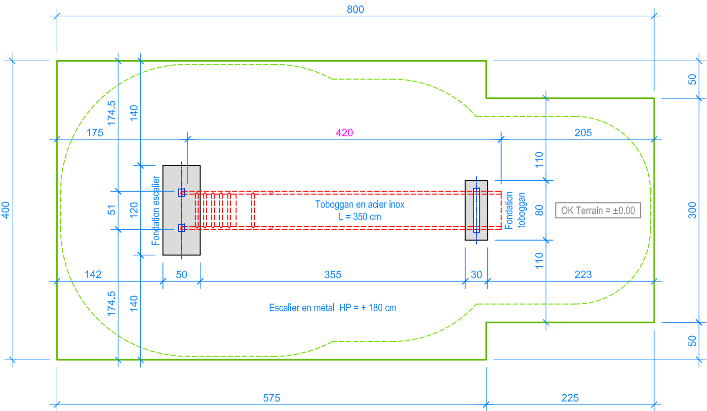
PLAN 1:50
