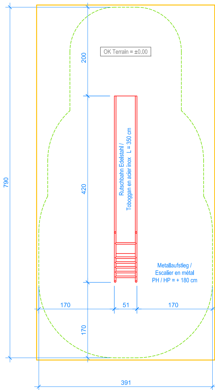
GRUNDRISS / PLAN 1:50
