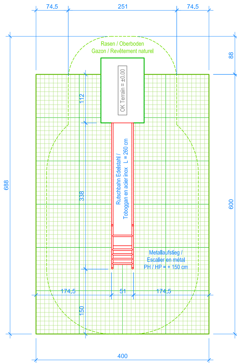
GRUNDRISS / PLAN 1:50
