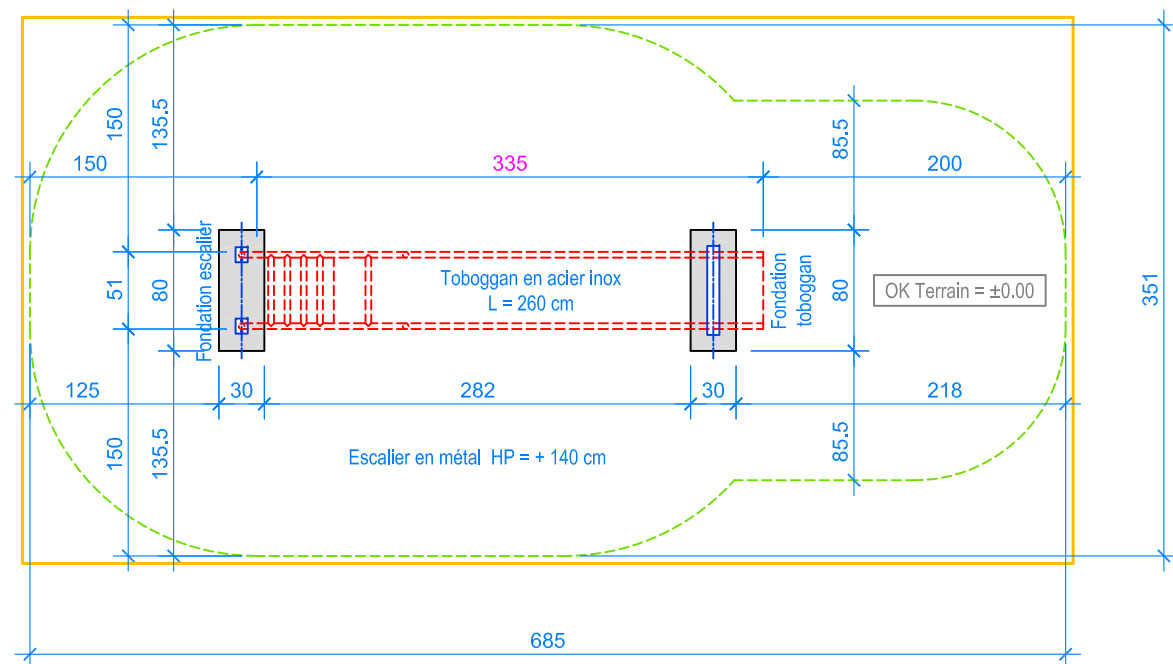
PLAN 1:50
