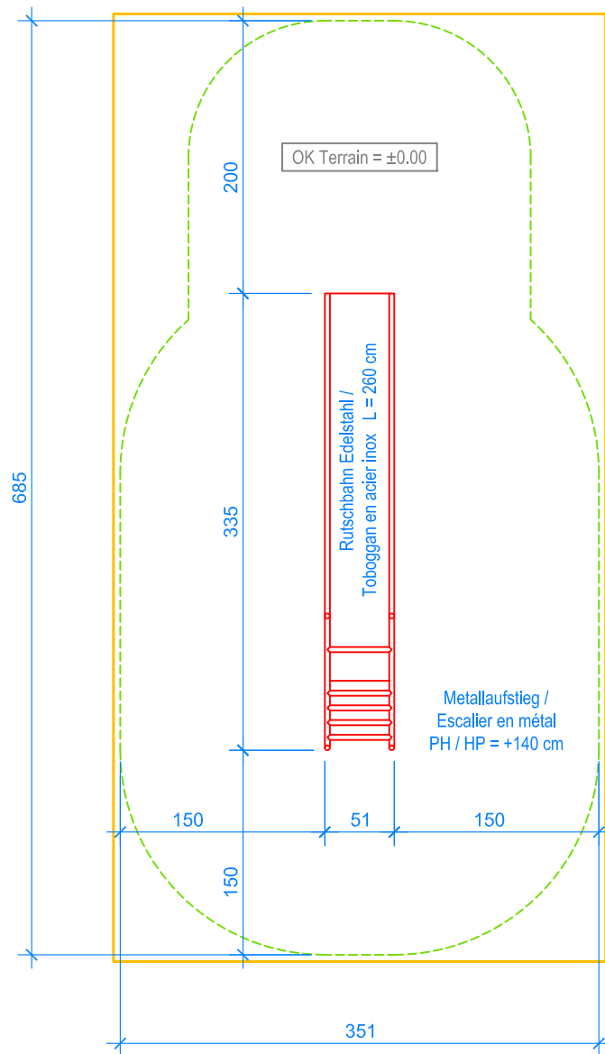
GRUNDRISS / PLAN 1:50
