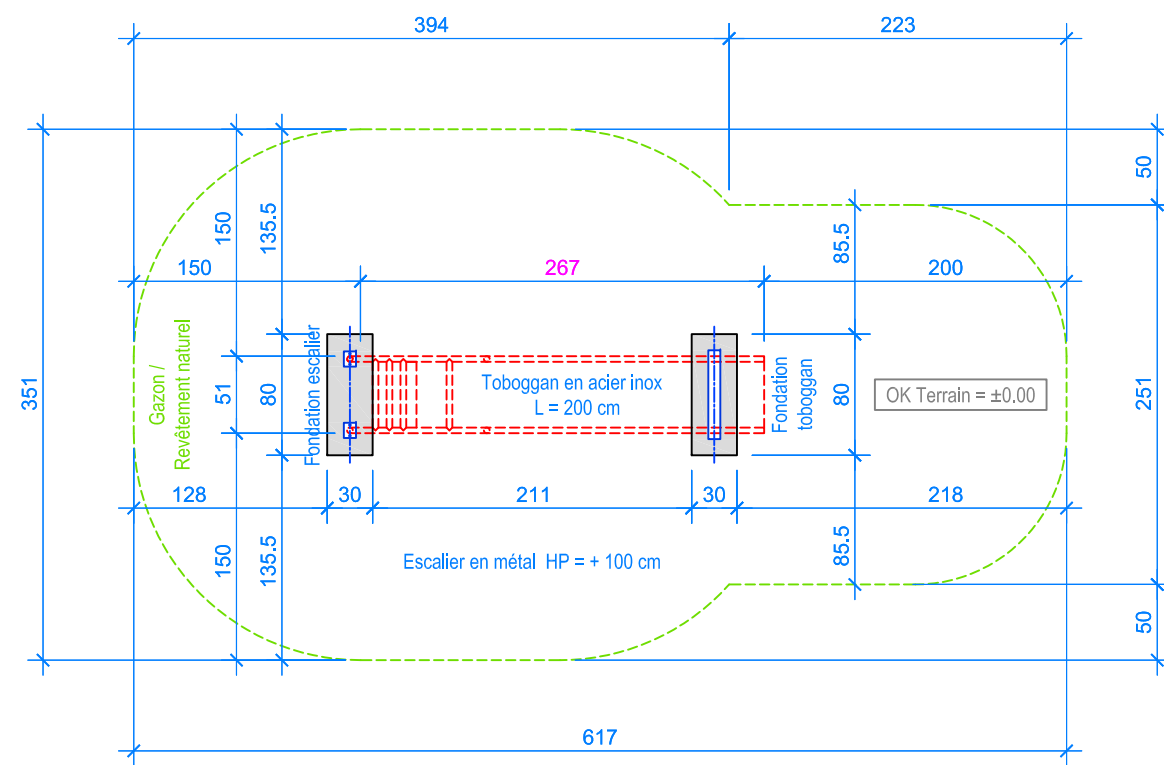
PLAN 1:50
