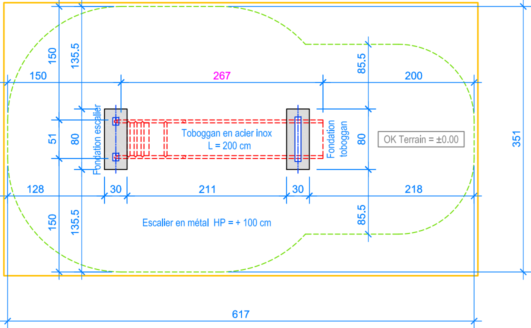
PLAN 1:50
