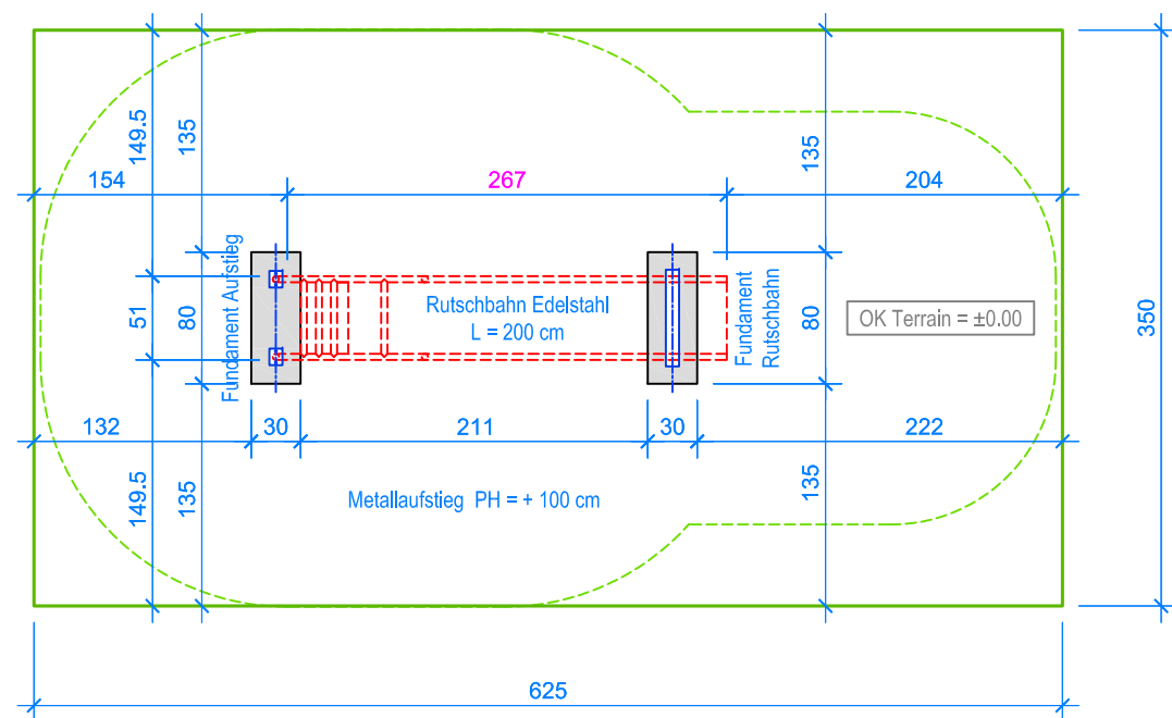
GRUNDRISS 1:50
