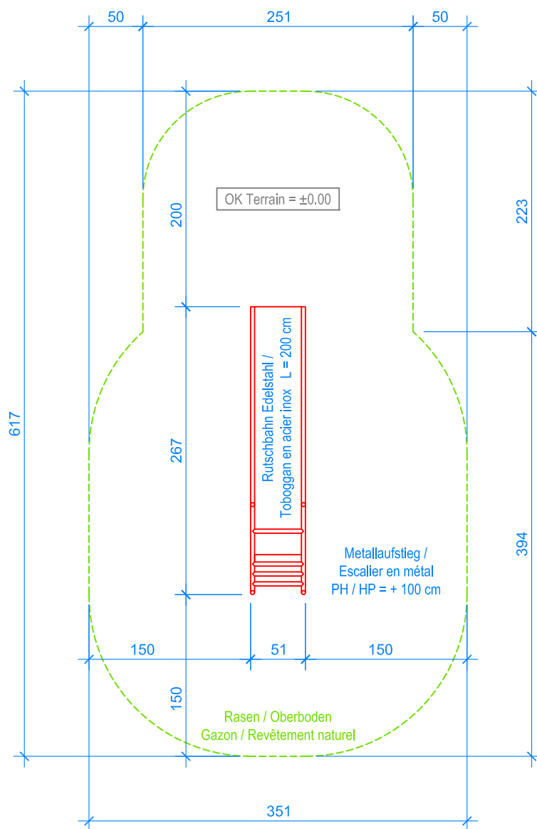
GRUNDRISS / PLAN 1:50
