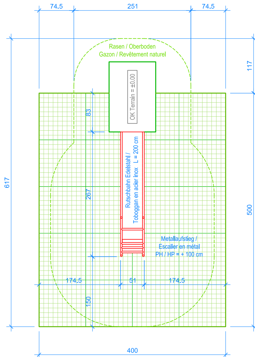
GRUNDRISS / PLAN 1:50
