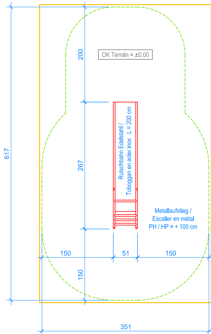
GRUNDRISS / PLAN 1:50
