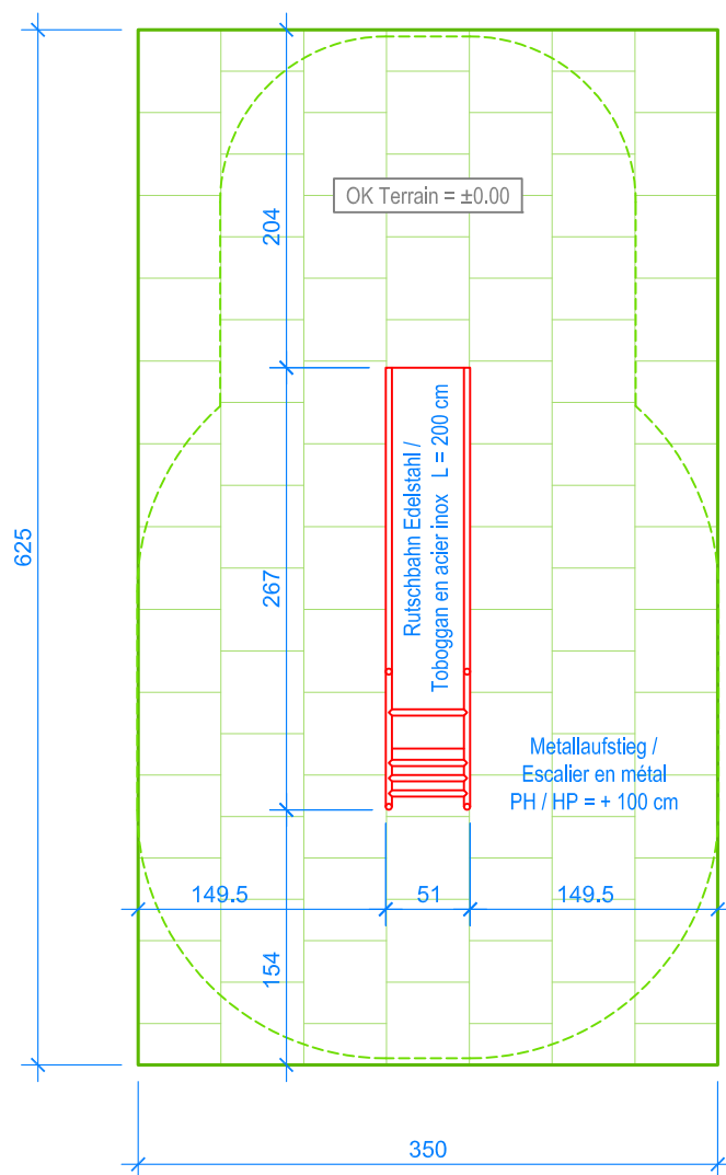
GRUNDRISS / PLAN 1:50
