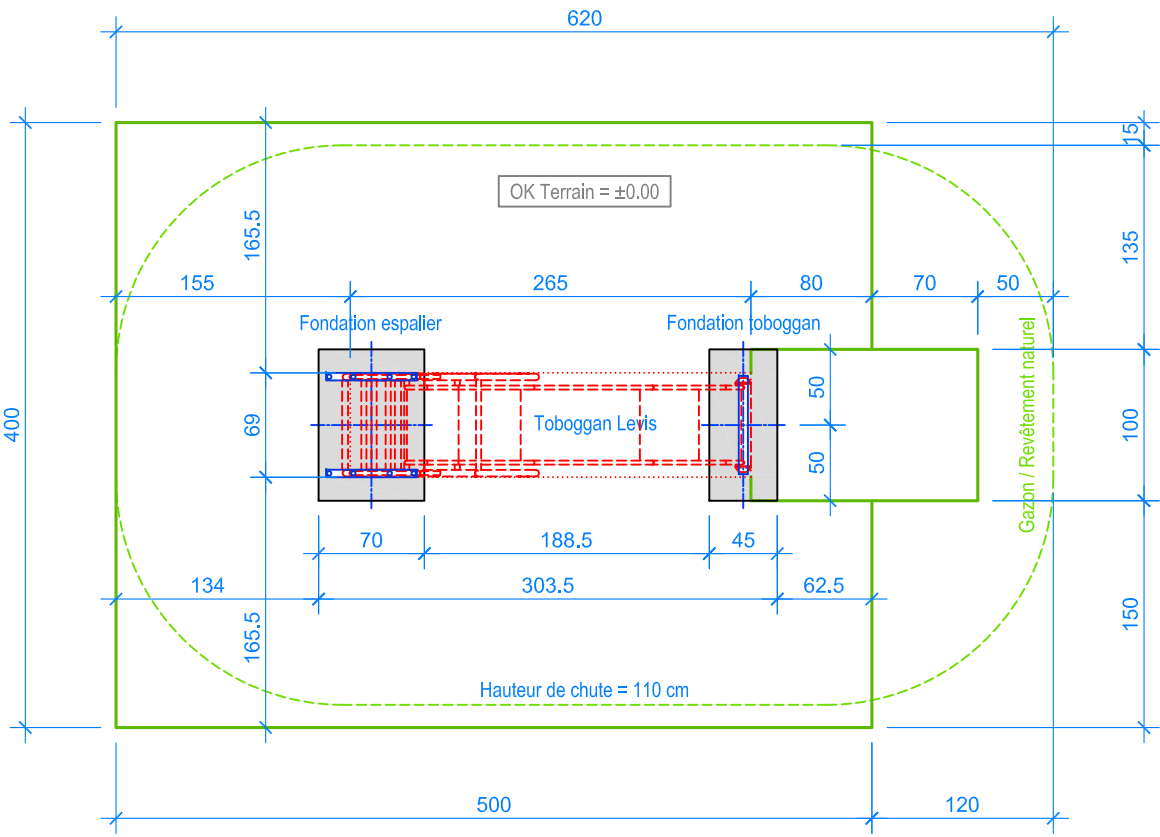
PLAN 1:50
