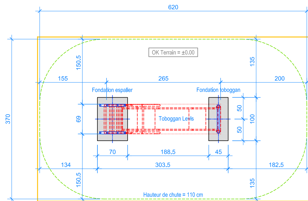
PLAN 1:50
