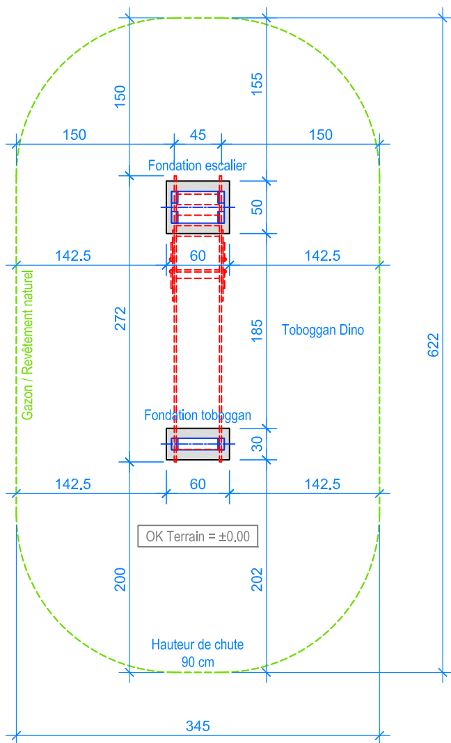
PLAN 1:50
