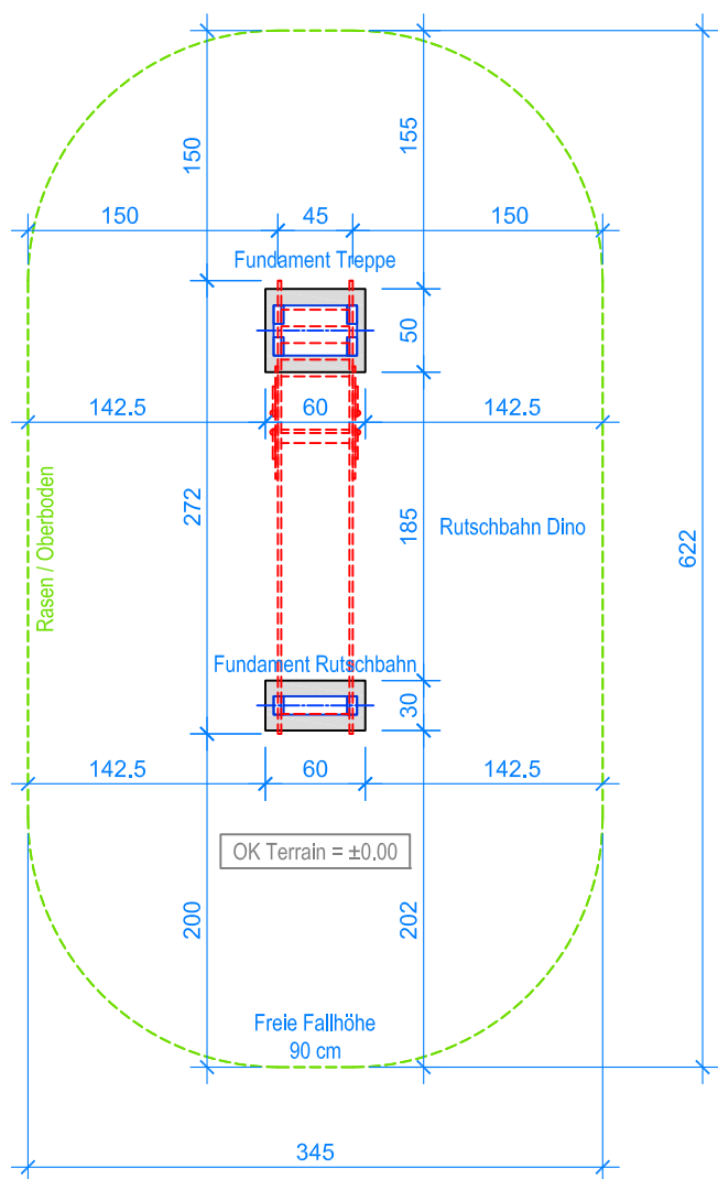
GRUNDRISS 1:50
