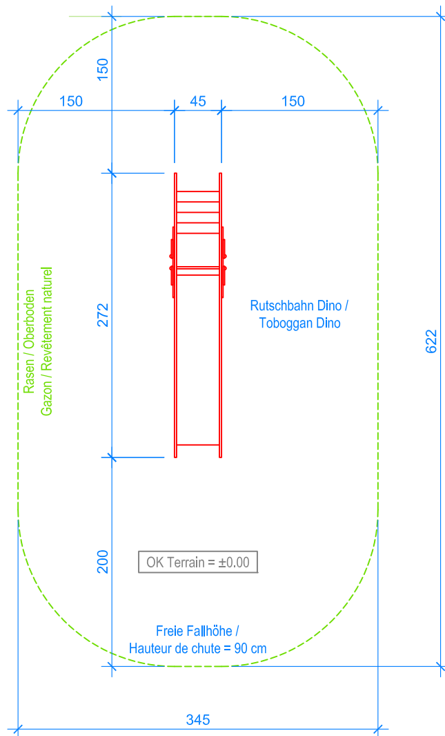
GRUNDRISS / PLAN 1:50
