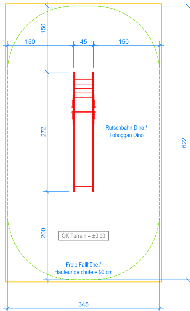
GRUNDRISS / PLAN 1:50
