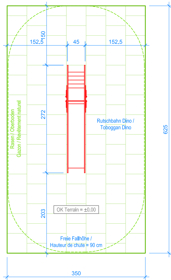
GRUNDRISS / PLAN 1:50
