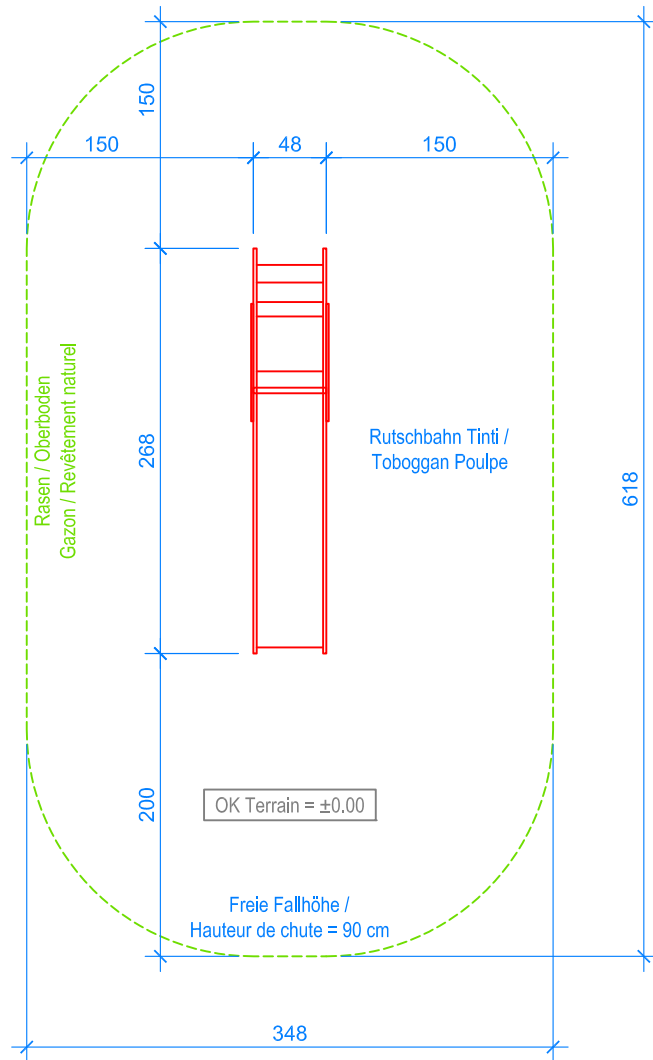
GRUNDRISS / PLAN 1:50
