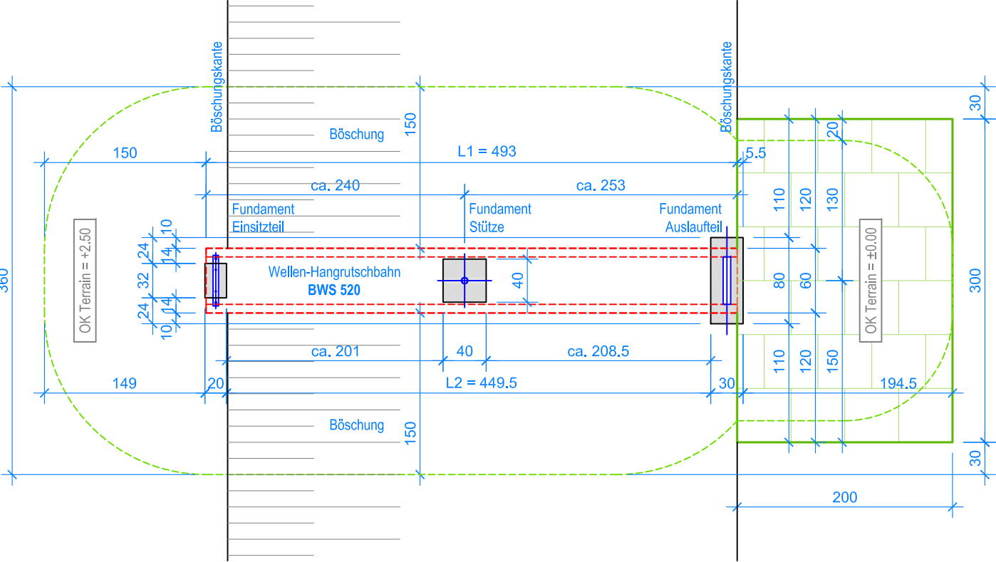
GRUNDRISS 1:50
