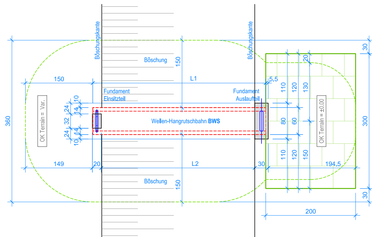
GRUNDRISS 1:50
