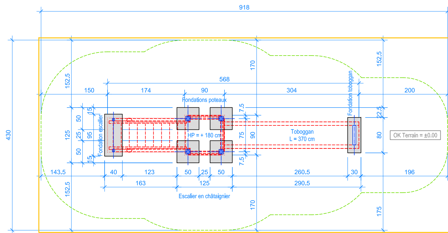
PLAN 1:50
