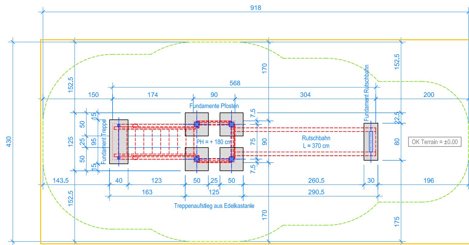
GRUNDRISS 1:50
