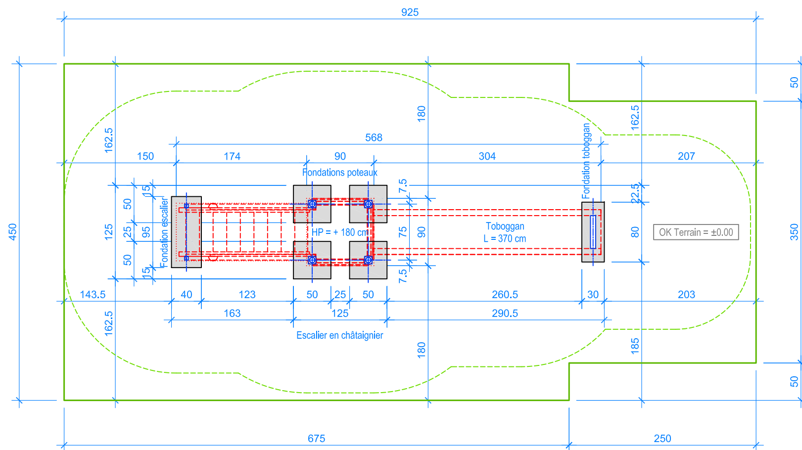
PLAN 1:50
