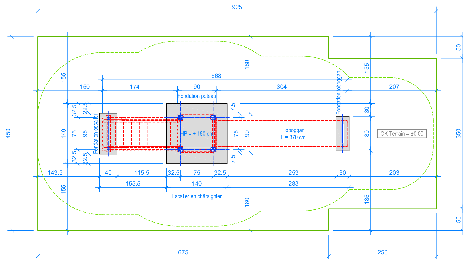
PLAN 1:50
