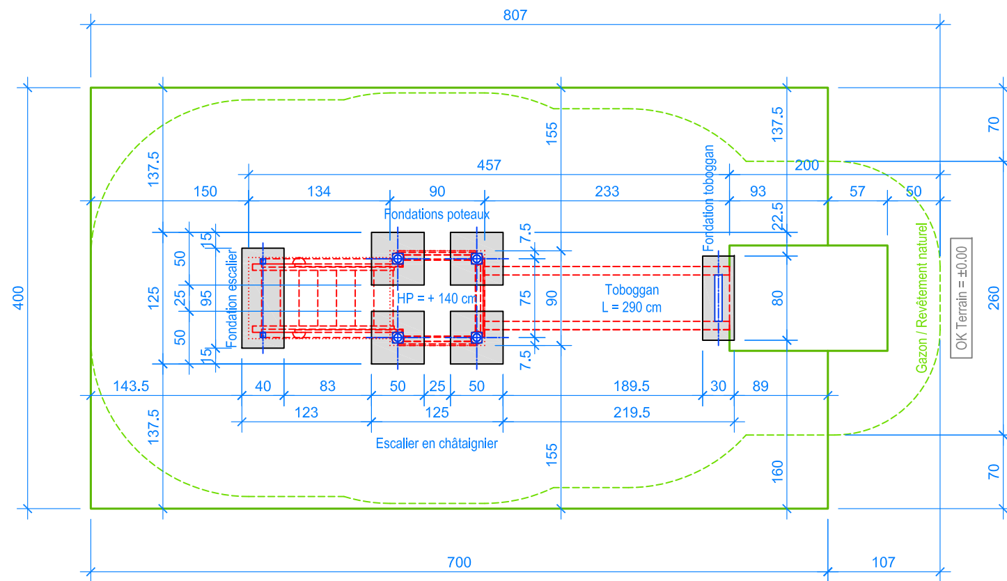
PLAN 1:50
