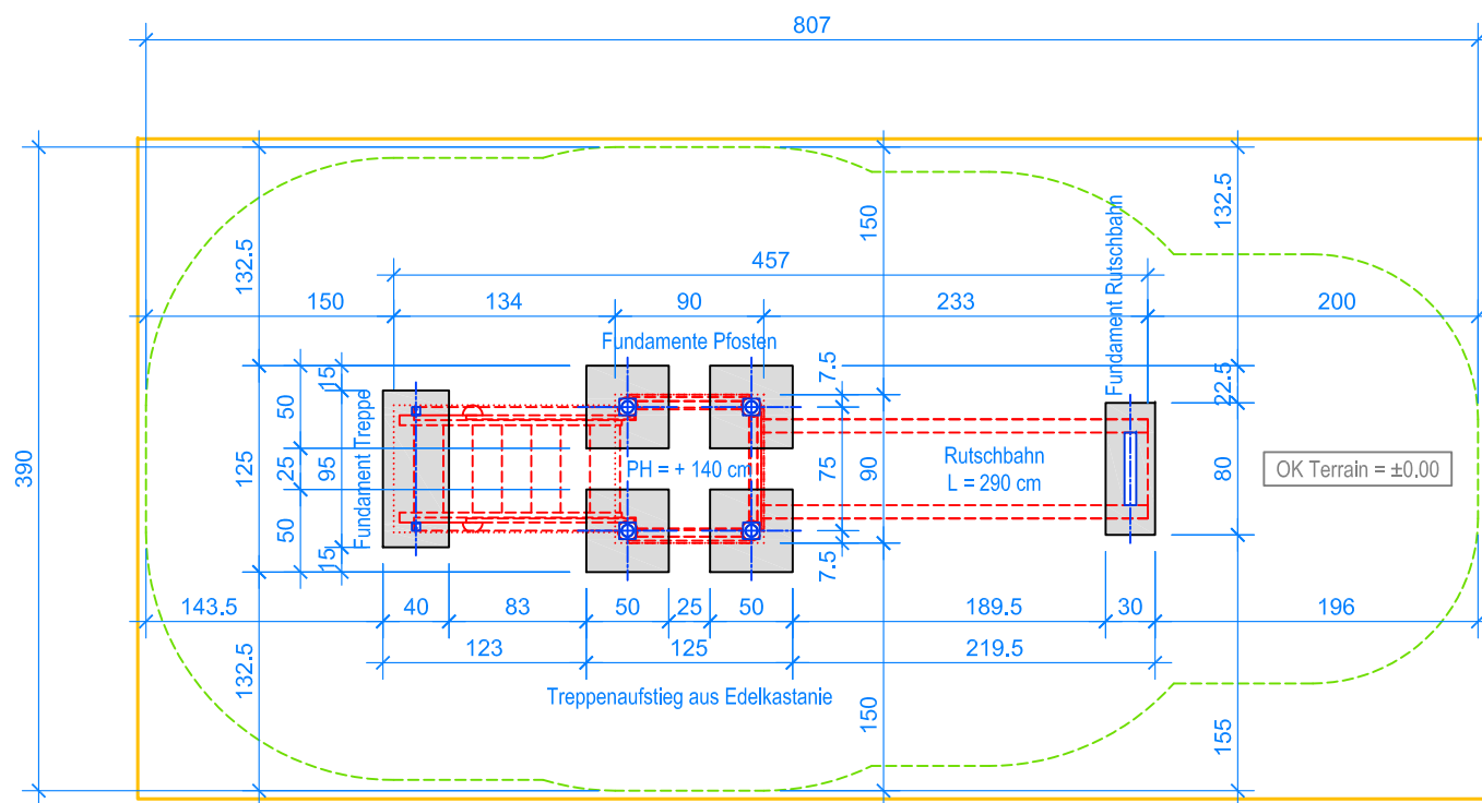
GRUNDRISS 1:50
