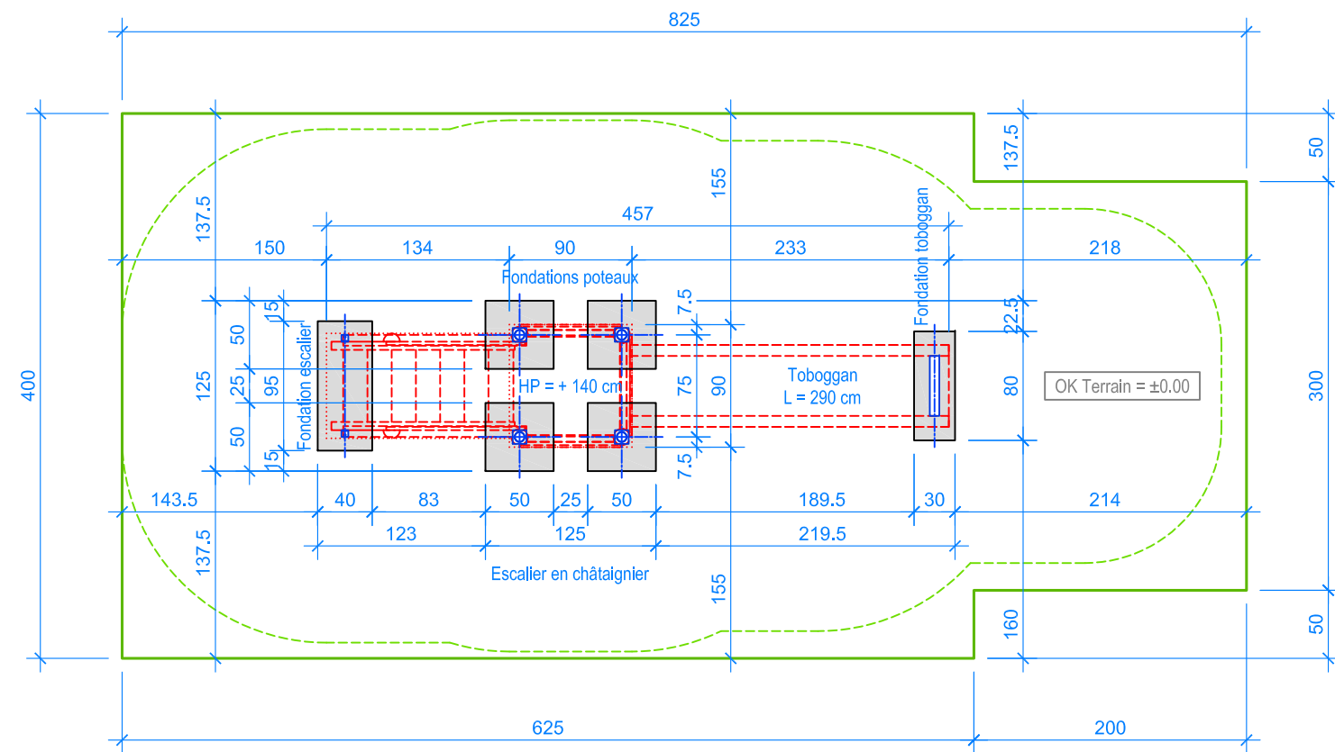
PLAN 1:50
