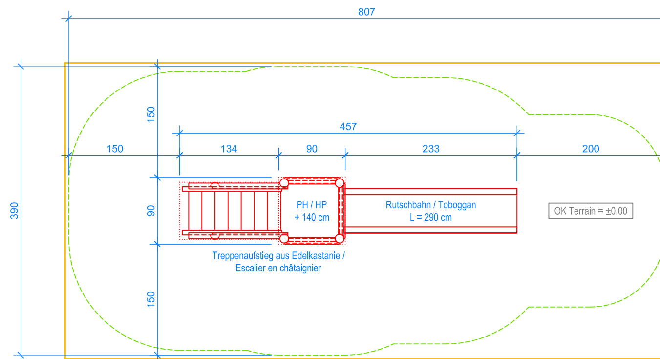
GRUNDRISS / PLAN 1:50
