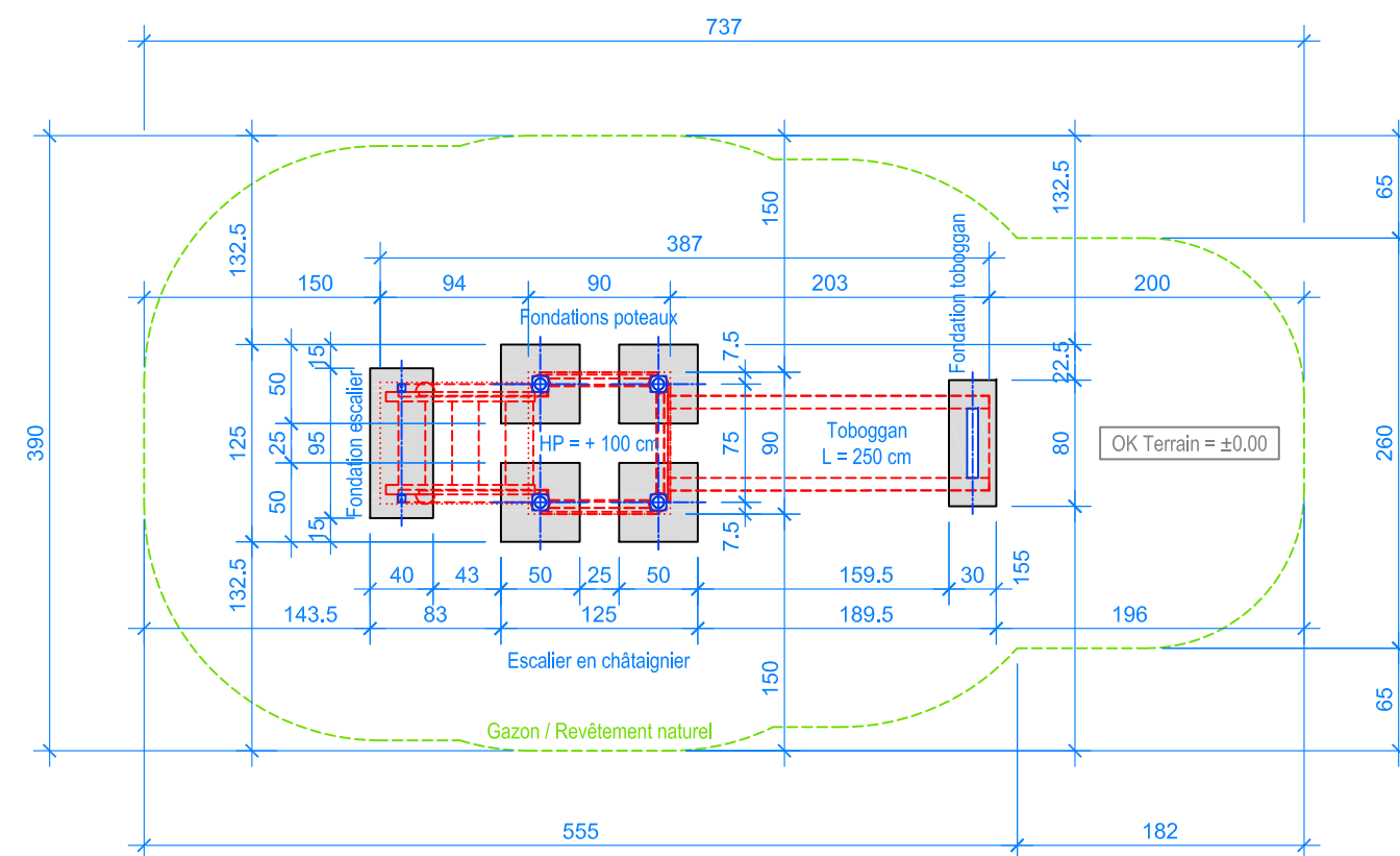
PLAN 1:50
