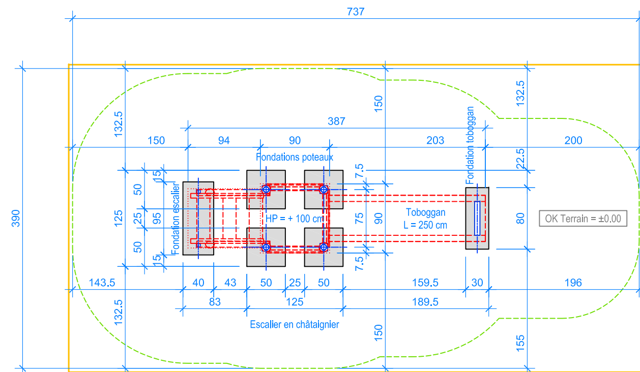
PLAN 1:50
