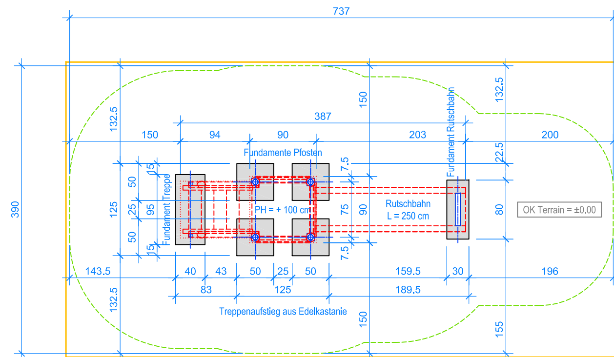
GRUNDRISS 1:50
