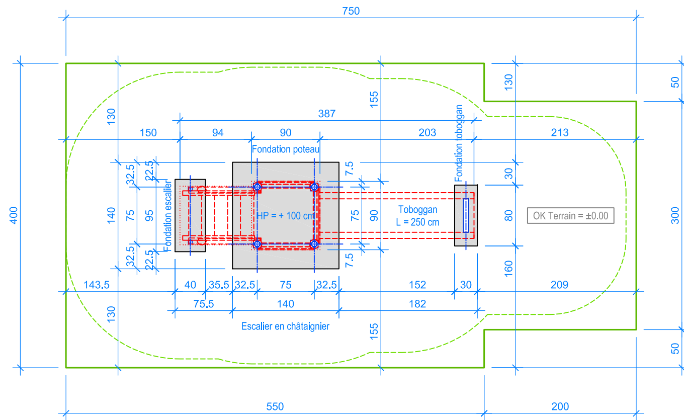
PLAN 1:50
