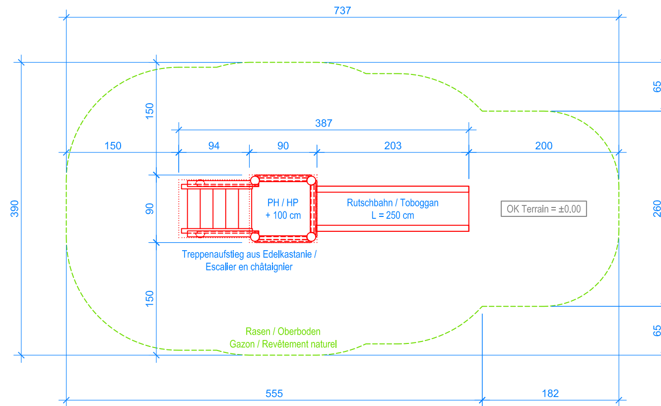
GRUNDRISS / PLAN 1:50
