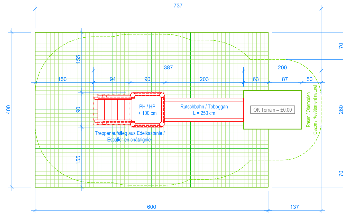
GRUNDRISS / PLAN 1:50
