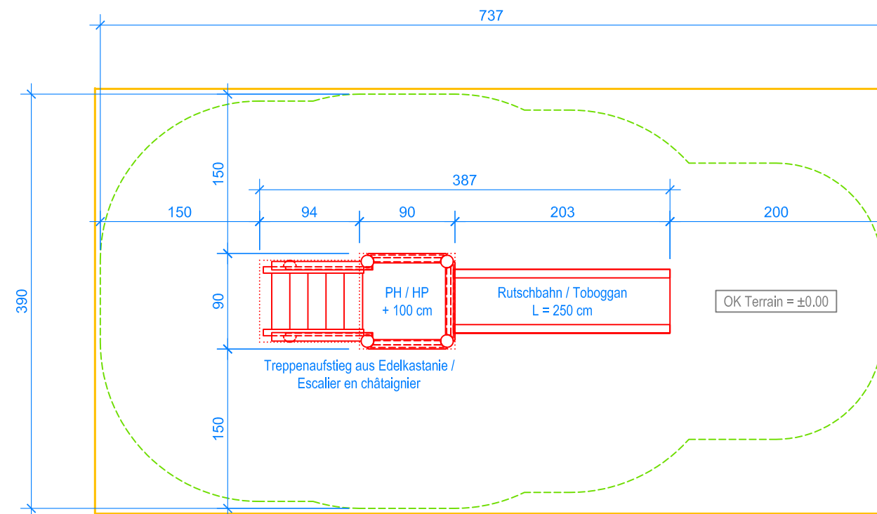
GRUNDRISS / PLAN 1:50
