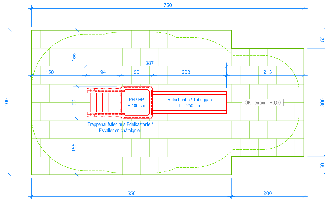
GRUNDRISS / PLAN 1:50
