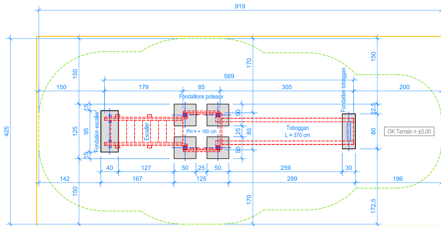
PLAN 1:50
