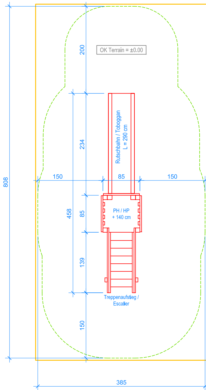
GRUNDRISS / PLAN 1:50
