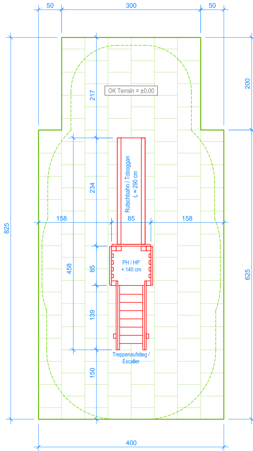
GRUNDRISS / PLAN 1:50
