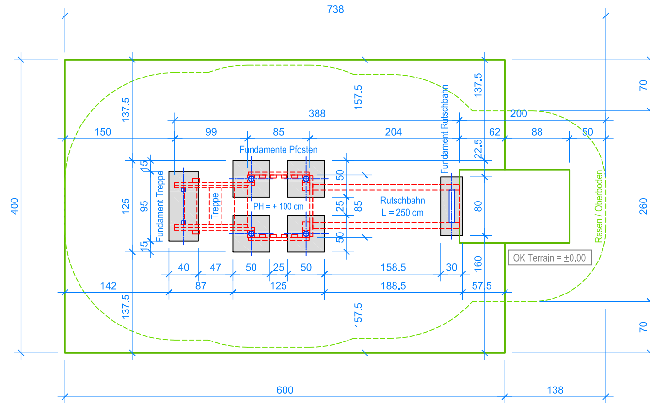
GRUNDRISS 1:50
