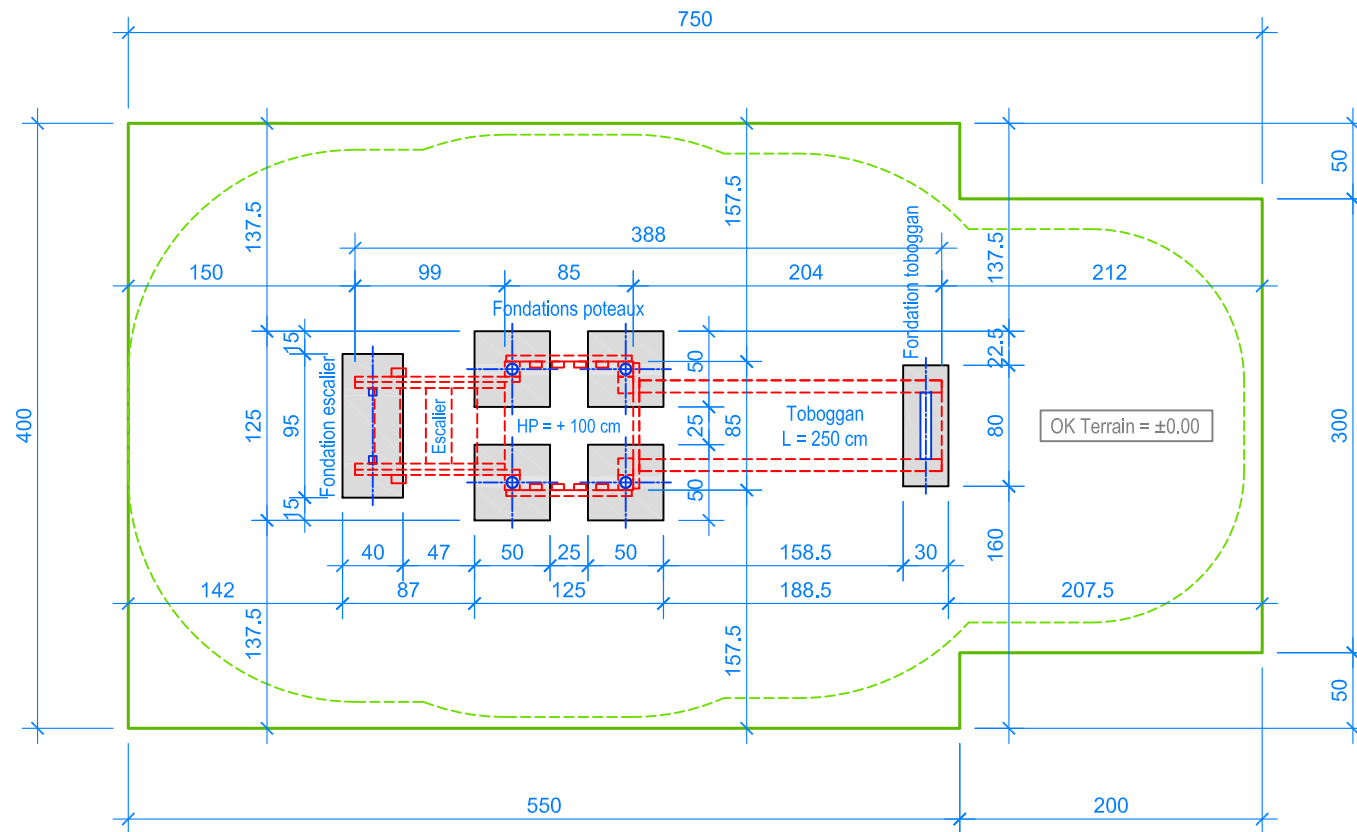
PLAN 1:50
