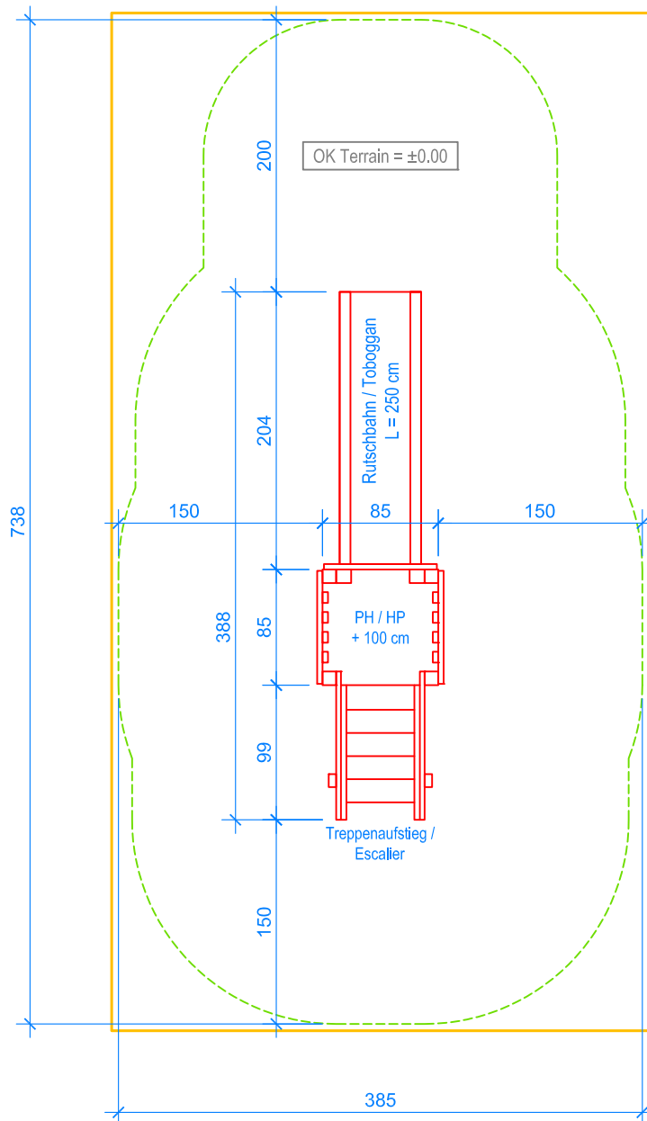
GRUNDRISS / PLAN 1:50
