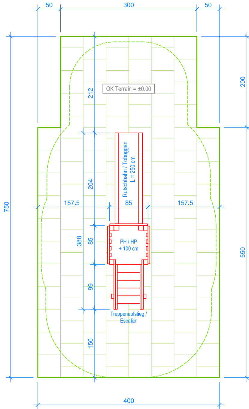
GRUNDRISS / PLAN 1:50
