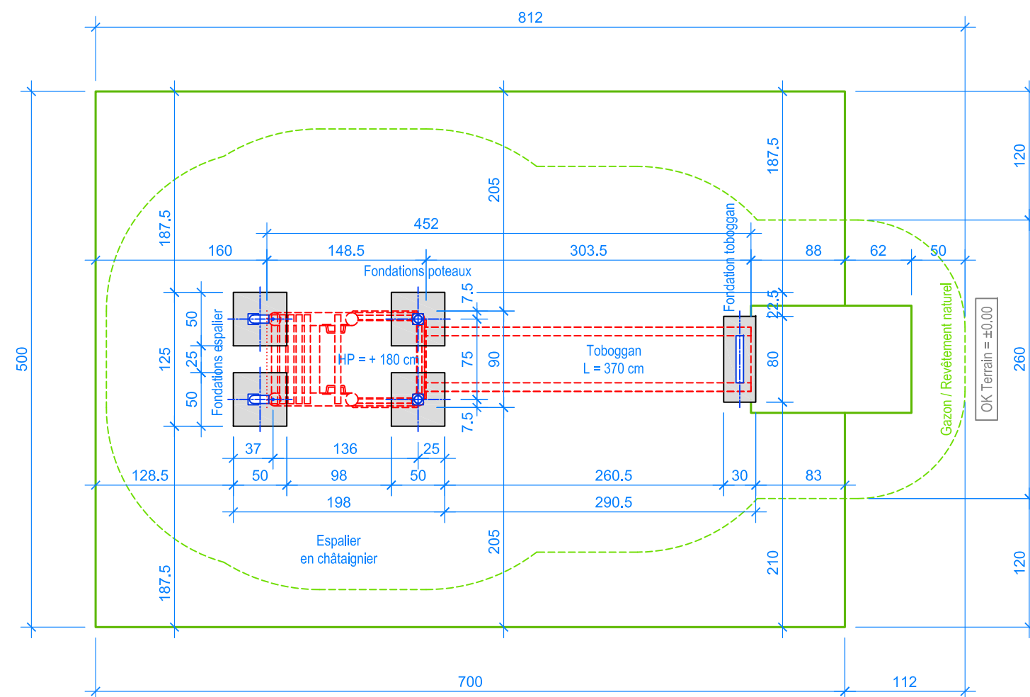
PLAN 1:50
