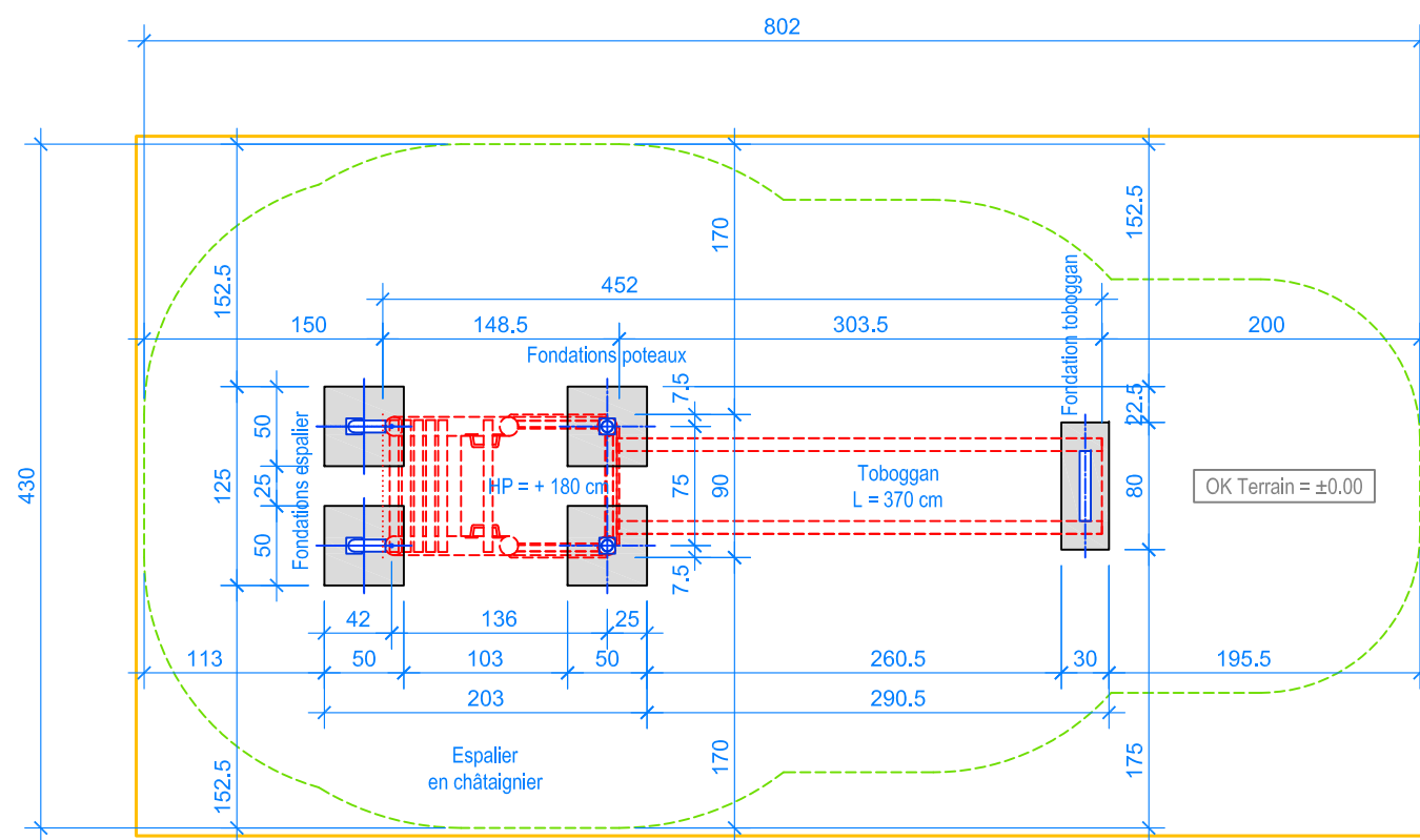
PLAN 1:50
