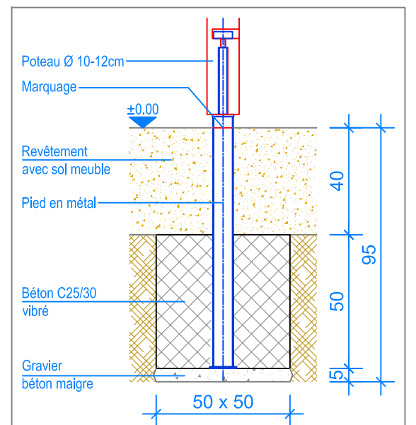
COUPE 1:20 FONDATION POTEAU
