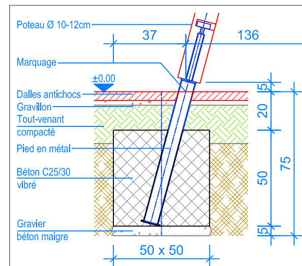
COUPE 1:20 FONDATION ESPALIER
