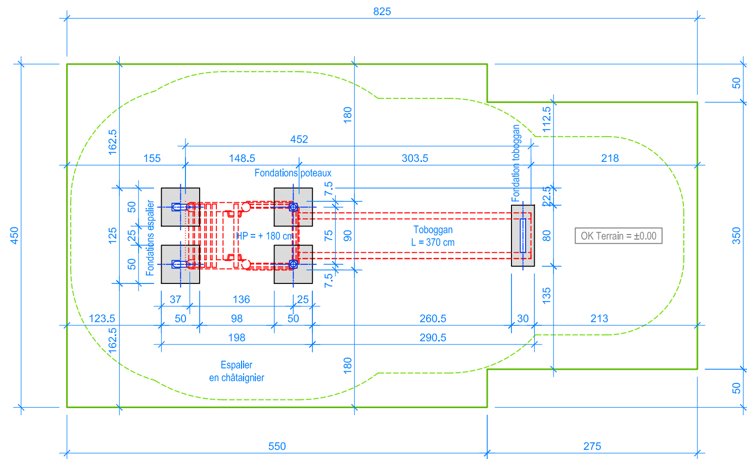
PLAN 1:50
