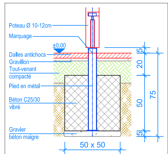
COUPE 1:20 FONDATION POTEAU
